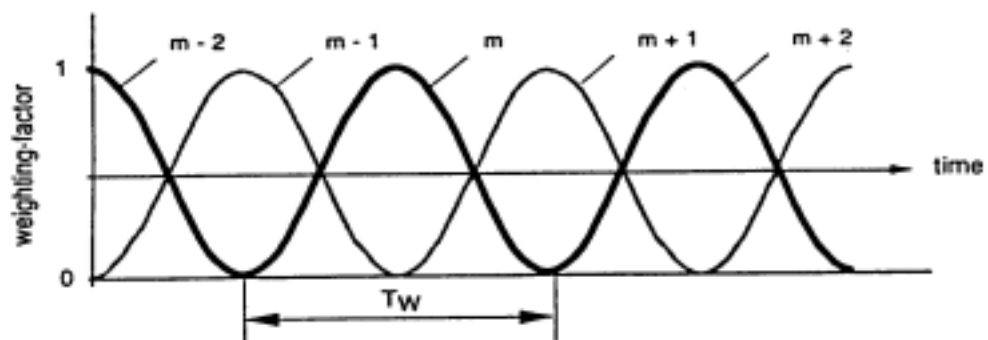
第7図 ハニングウインドの形態と配置
