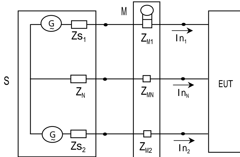
第4図 単相3線機器用測定回路
