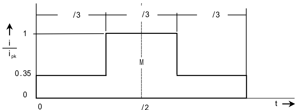
第2図 特殊な電流波形
