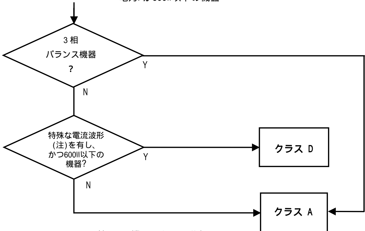
第1図 機器のクラス分類
