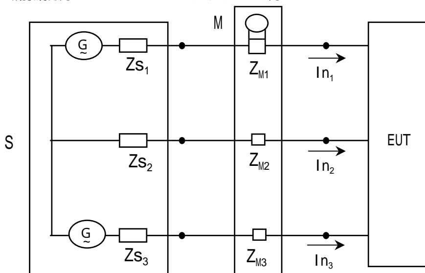
第5図 3相機器用測定回路
