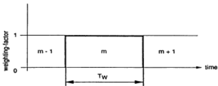
第6図 レクタングラーウインドの形態と配置
